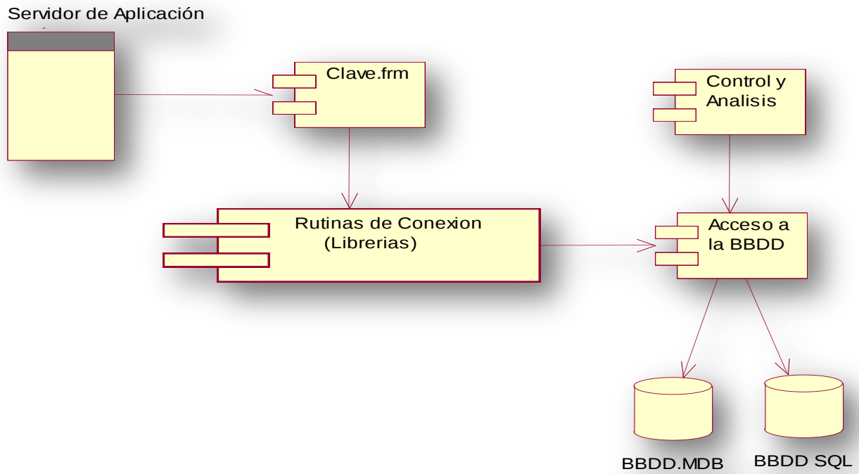
Figura 39: Diagrama Modelo de Componentes, detallado.
