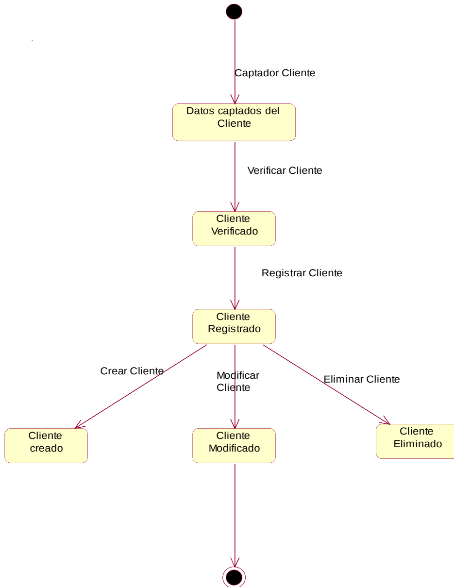
Figura10: Modelo Estado - Registro Cliente
