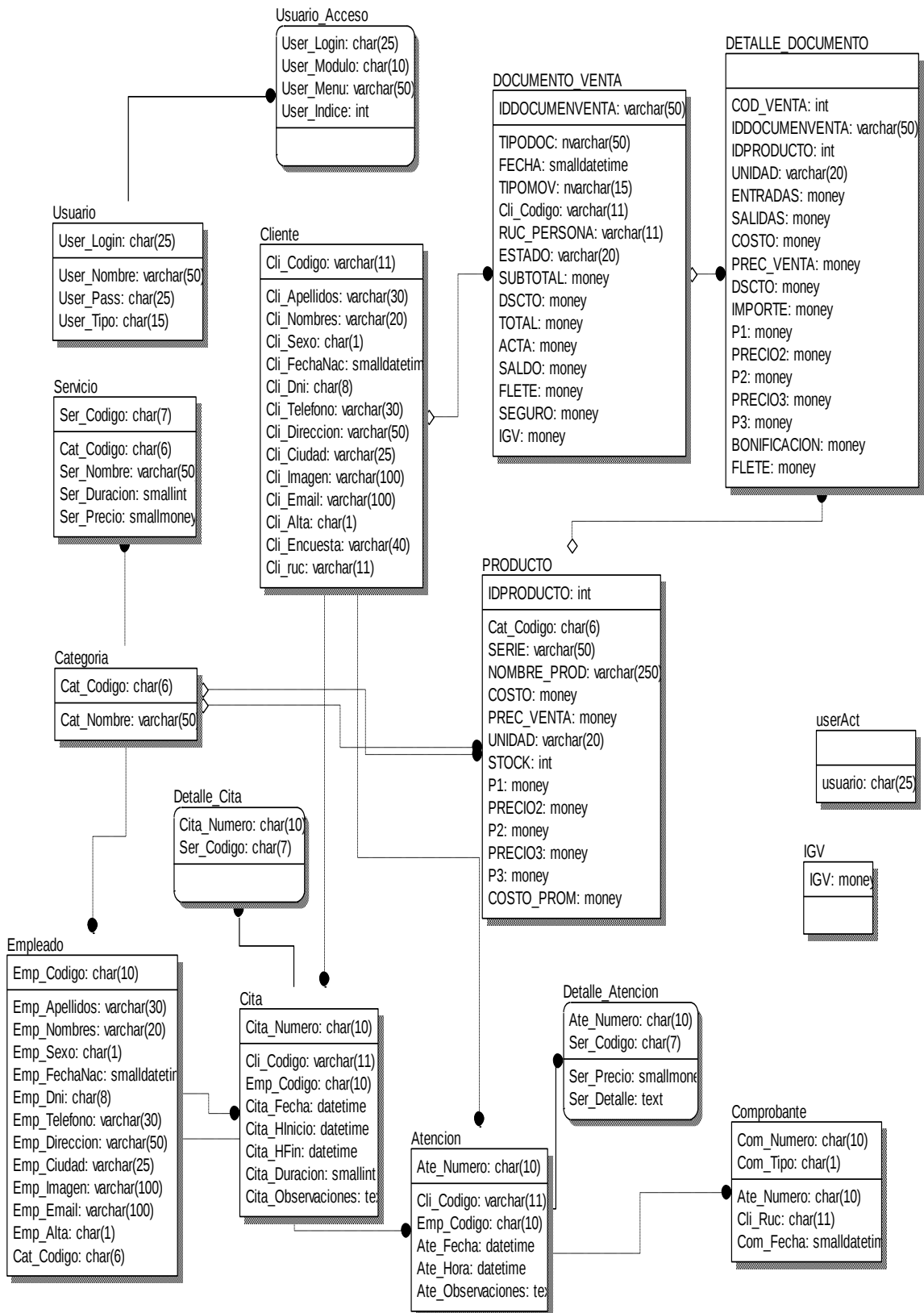
Figura 38: Modelo Físico - Muestra el diseño de la base de datos
