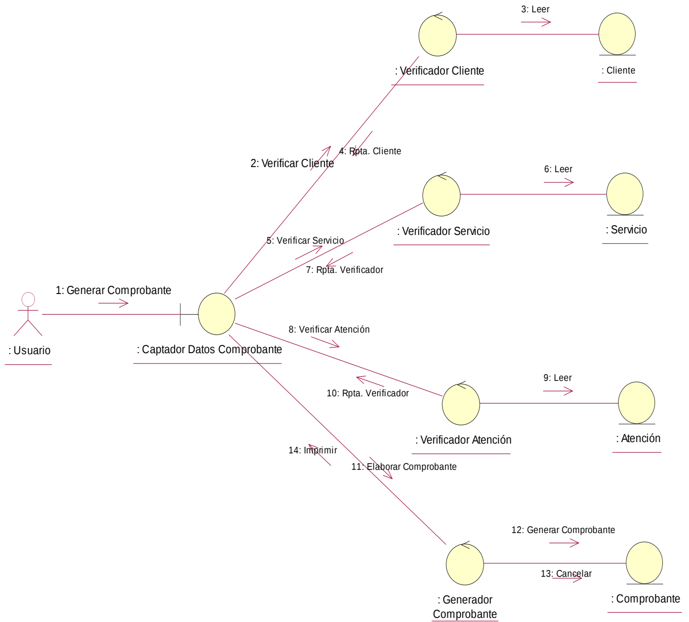
Figura 23: Diagrama de colaboraciones - Generar comprobante
