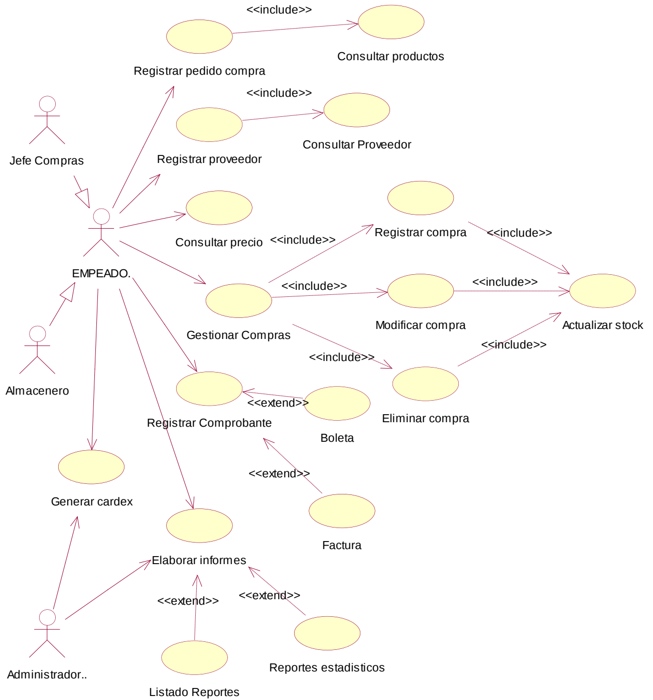
Figura 08: Caso de uso proceso Gestionar Compras
