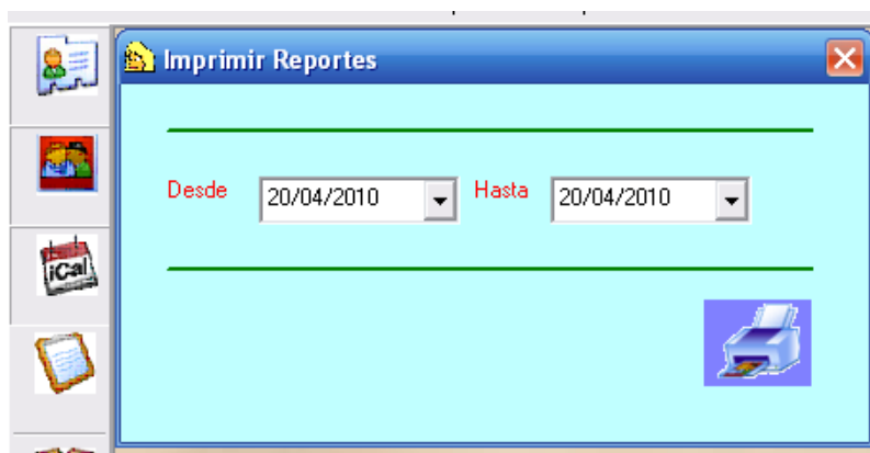
Fig.62: Formulario Reportes
