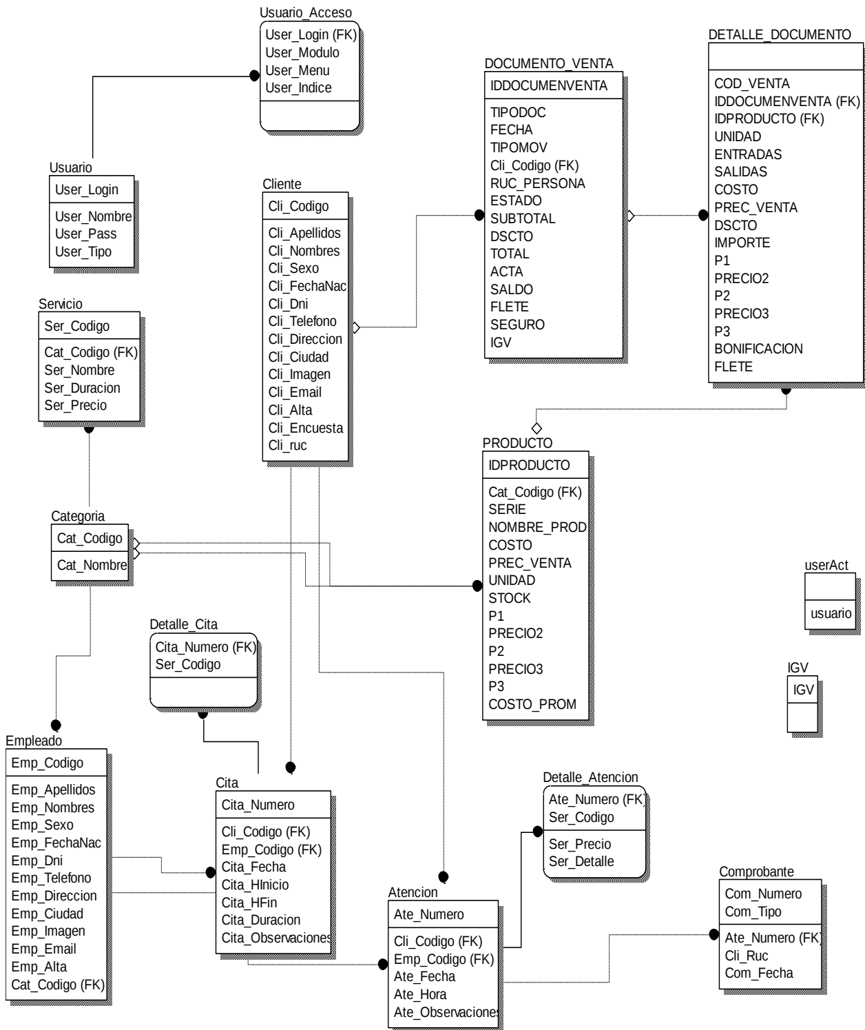
Figura 37: Modelo Lógico - Muestra el diseño de la base de datos
