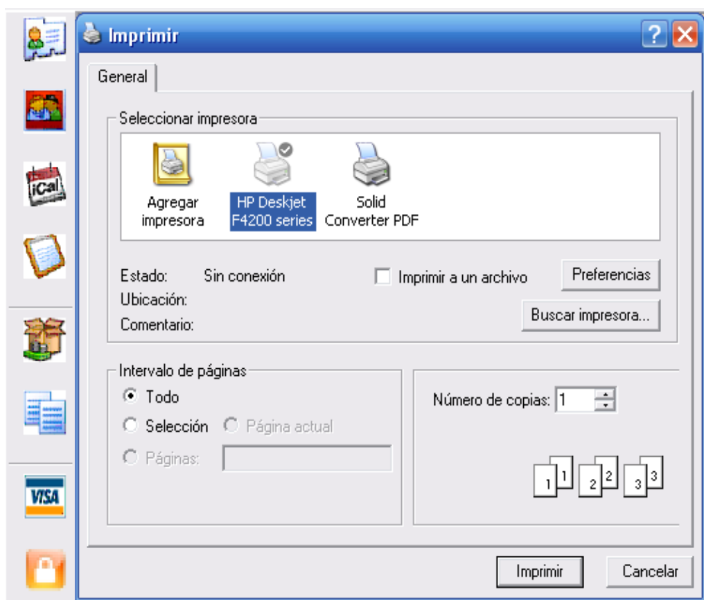
Fig.61: Configurar Impresora
